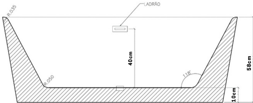
CORTE 01
