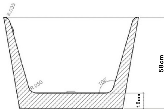
CORTE 02
